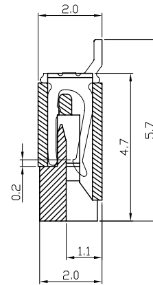
SECTION A-A 下接触
